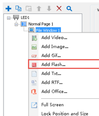
Fig. 5-7 Add Flash
